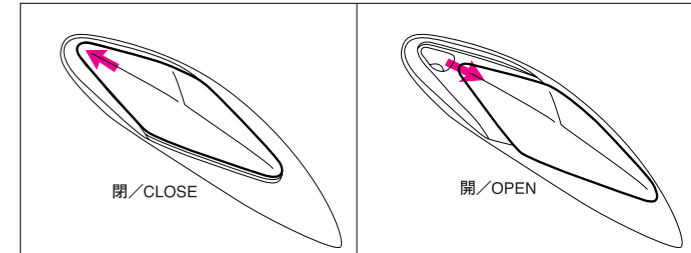
STエア アウトレット ST Air Outlet
