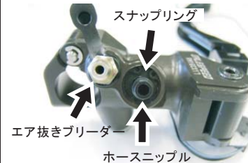
ホースニップル
